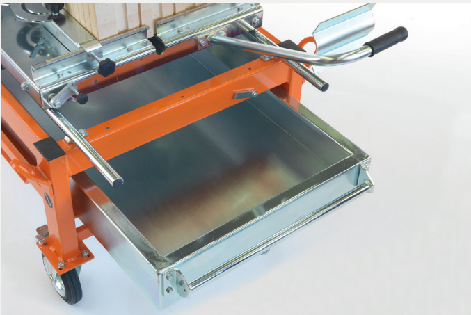
Ausziehbare Wasserwanne.
