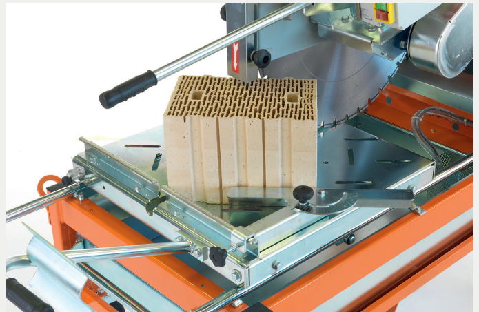
Winkelanschlag 0–180°.
