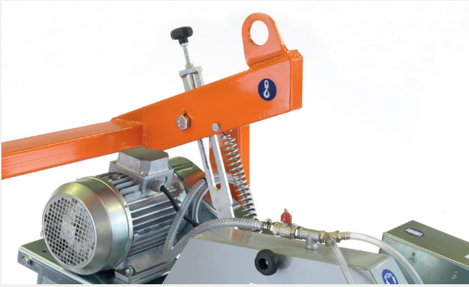
Ein zentraler Kranhaken. Motor mit elektrischer Bremse sichert das rasche Anhalten der Diamanttrennscheibe.
