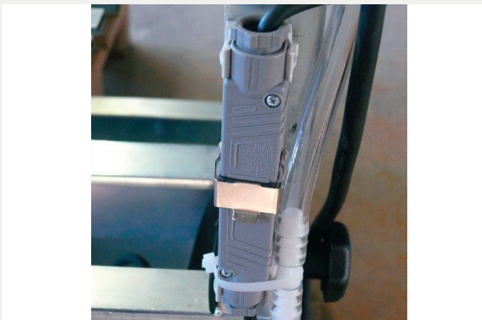
Steckbare Wasserpumpe für ein rasches und sicheres Auswechseln der Wasserpumpe.
