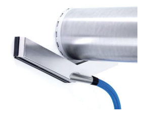
Wassersammel- vorrichtung für das Kernbohren, V-förmiger Sammel- körper max. D: 350 mm
