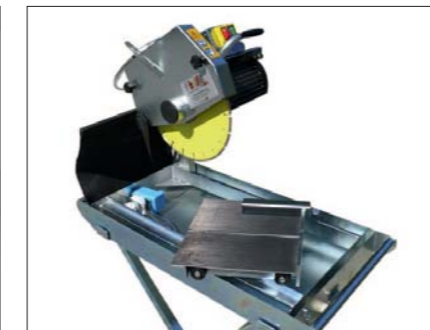
Hohe Beweglichkeit des Wippkopfes ermöglicht eine höhere Schnitttiefe im Umdrehschnitt bis ca. 160 mm.
